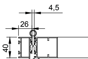
Unidad sin tapajuntas
