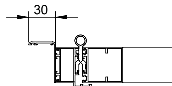
Unidad con tapajuntas
